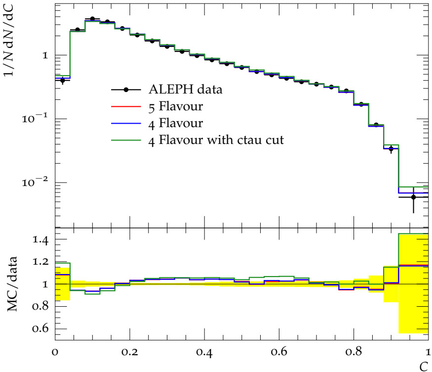
C parameter (charged)
