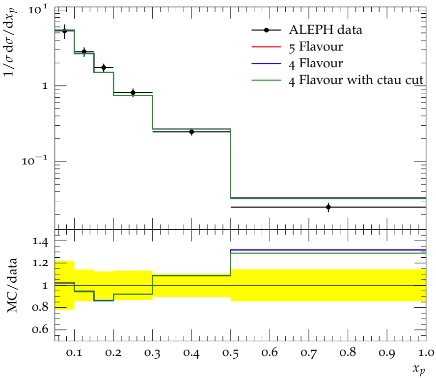
\omega(782) spectrum
